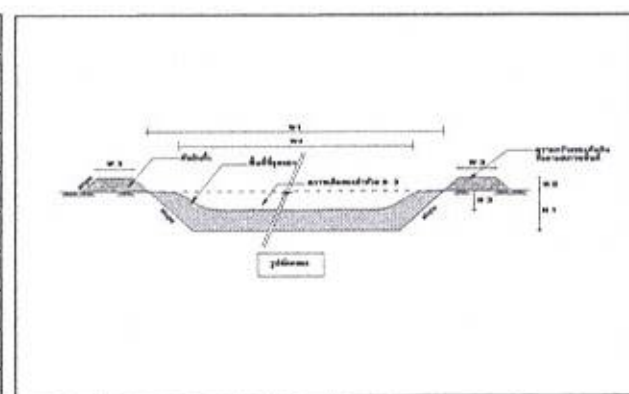
รูปตัด STA. 0+170
