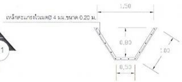
รูปตัด A1
