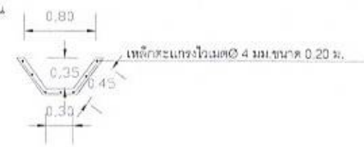
รูปตัด A2
