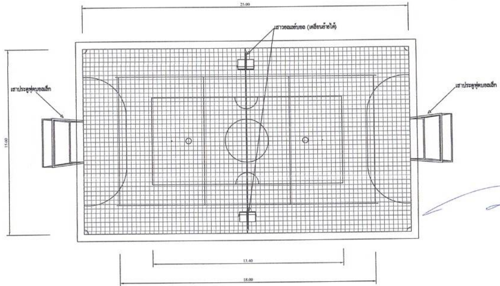
แบบสนามกีฬากลางแจ้งเอนกประสงค์ ขนาดกว้าง 15 เมตร x 25 เมตร
